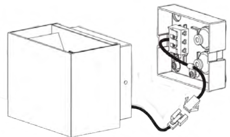
EASYbase für einfache Montage
