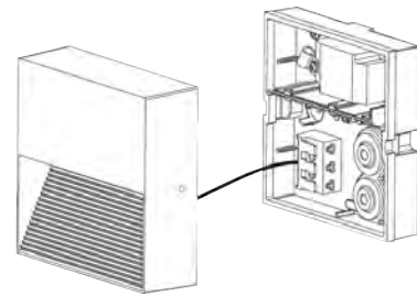
EASYbase für einfache Montage
