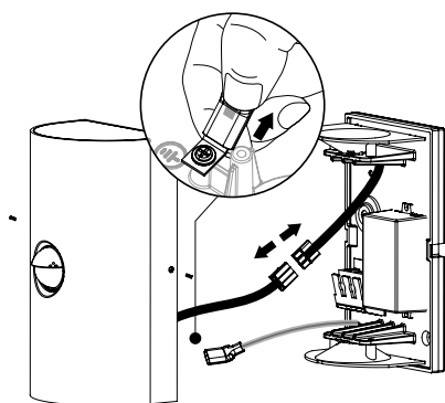
EASYbase für einfache Montage mit doppeltem Kabeleinlass.
