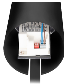
Bequeme Einstellung der Leistung am Netzteil
