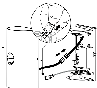
EASYbase für einfache Montage mit doppeltem Kabeleinlass.
